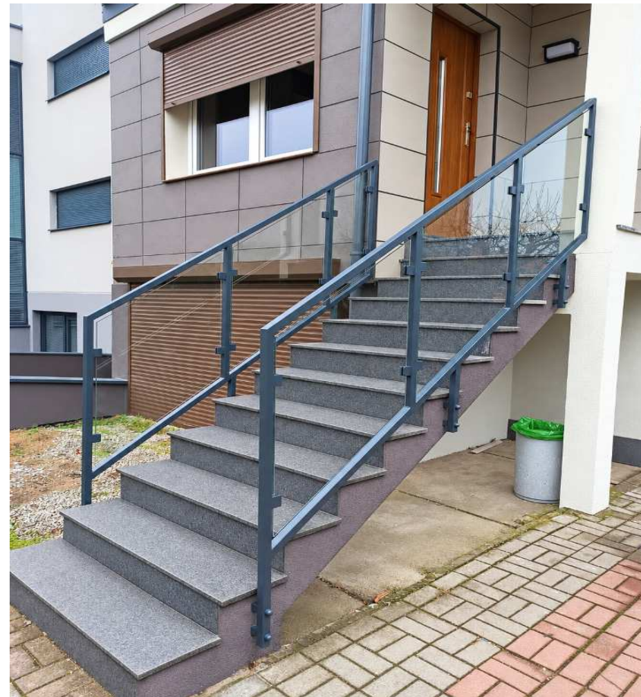
Szkło w ramie na uchwytych
