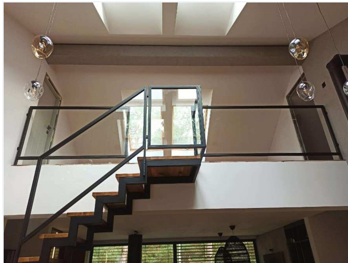
Szkło w ramie z dociskiem
